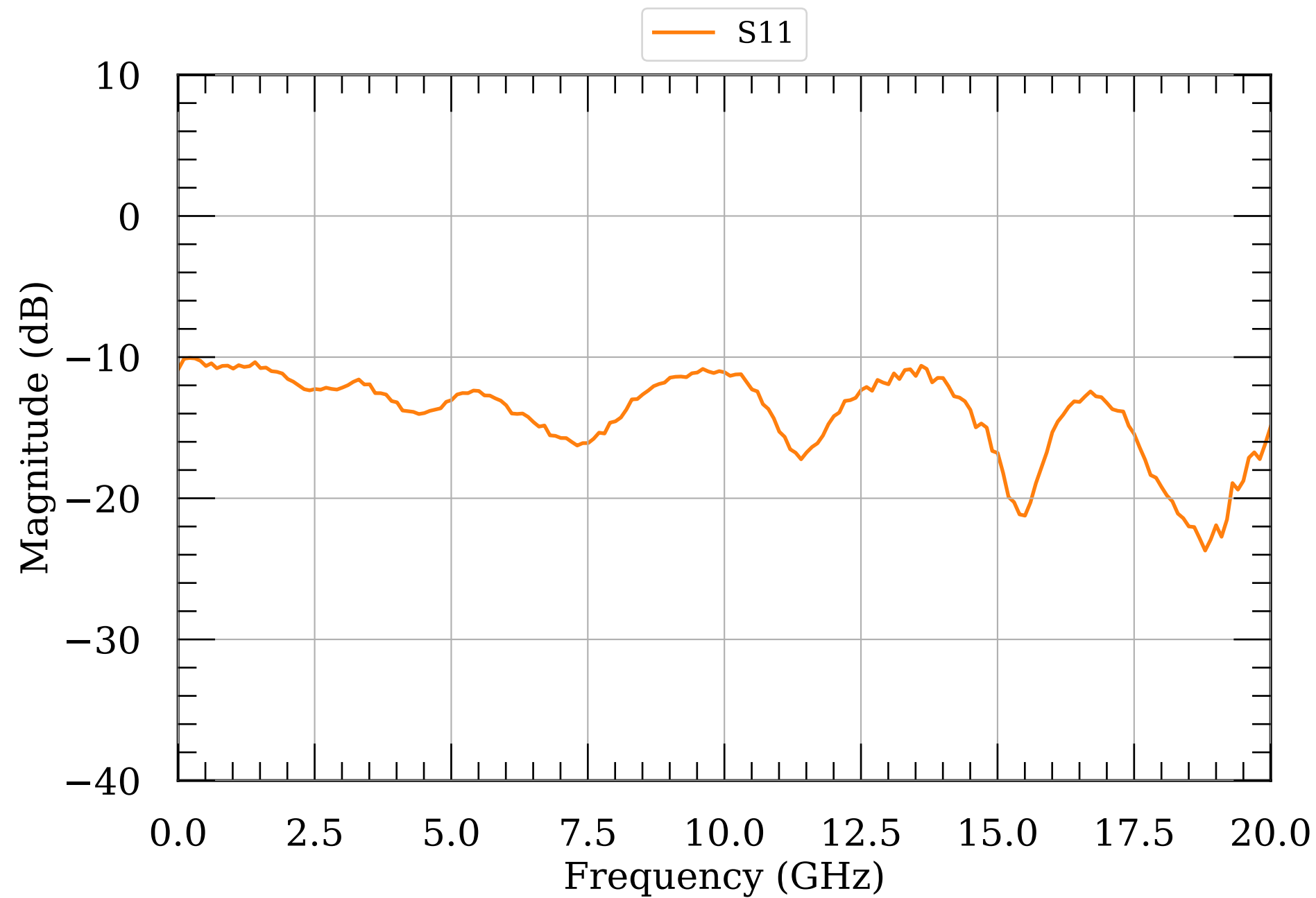
LNA S-params module050
